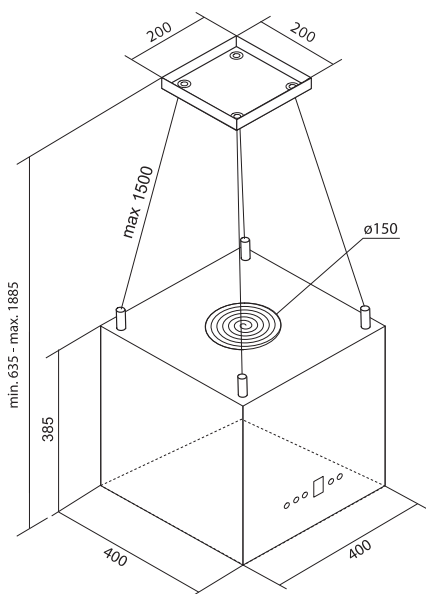
Okap OK-4 SANDY MINI
