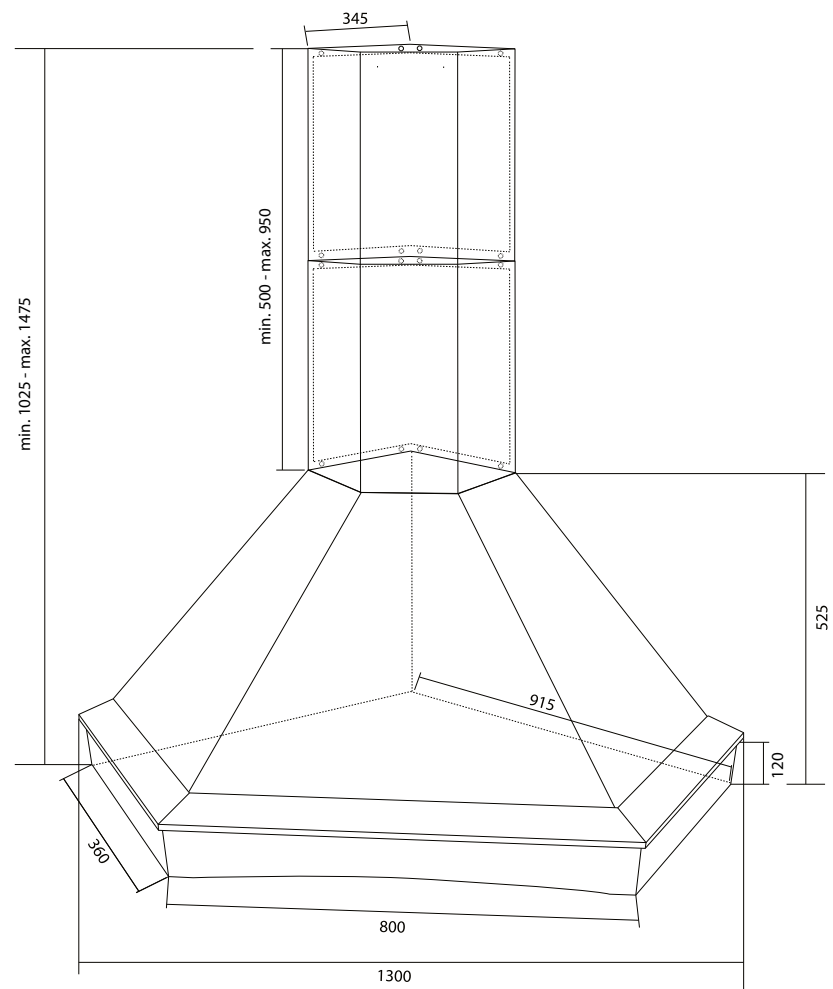
Okap OK-3 NAROŻNY
